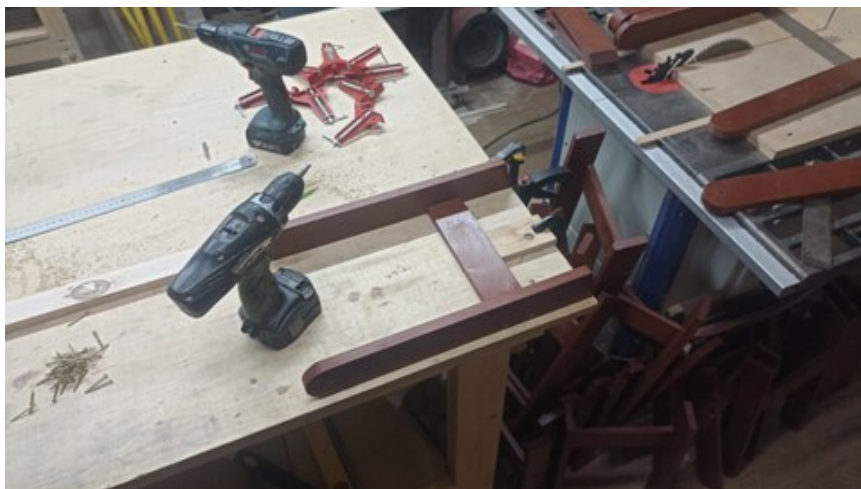
процесс изготовления деревянных раскладных скамеек
